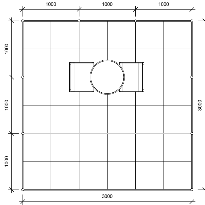
① PLAN LAYOUT 1 : 25
